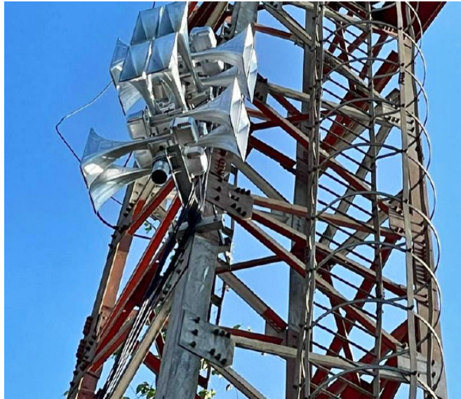
जीआई टावरों पर सायरन लगाया गया
